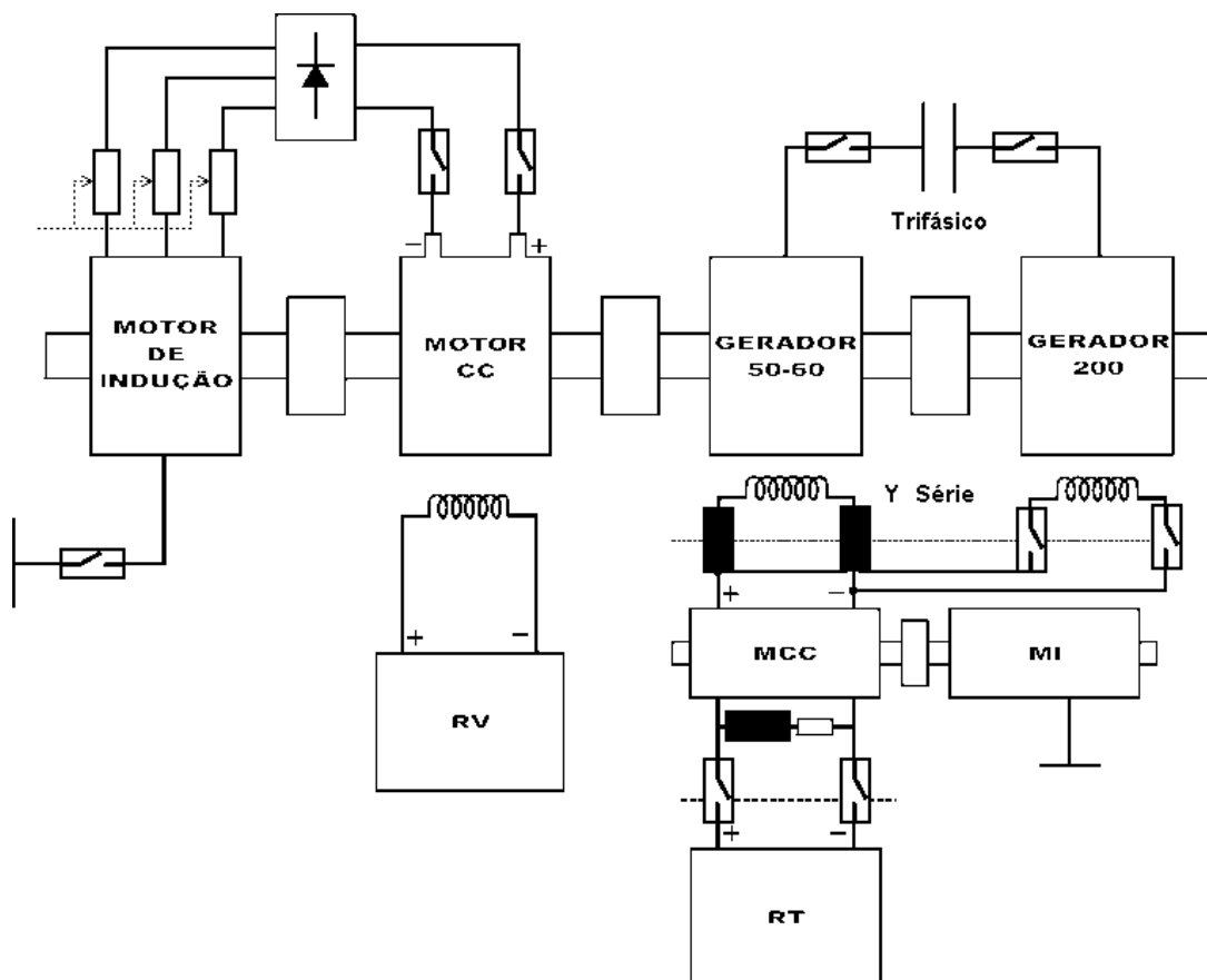
FIGURA 1 - Configuração básica das unidades.
