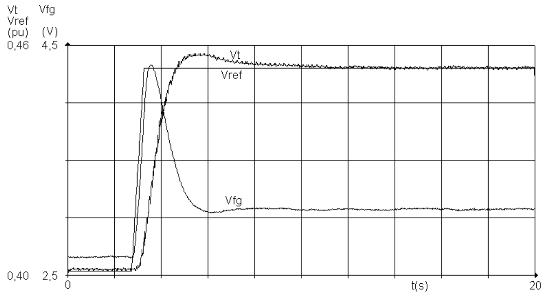
FIGURA 14 - Resposta ao Degrau no Regulador de Tensão.
