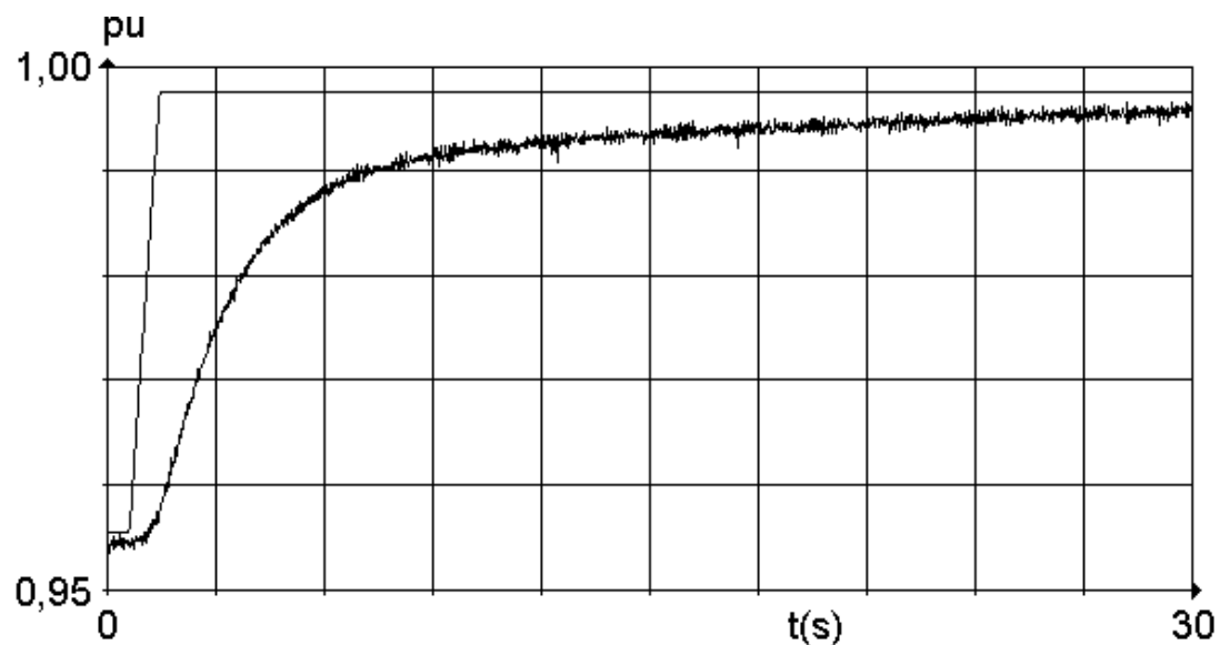
FIGURA 11 - Resposta ao degrau na referência de velocidade.
